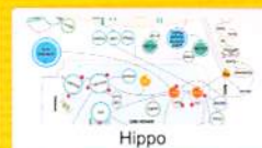
Hippo
